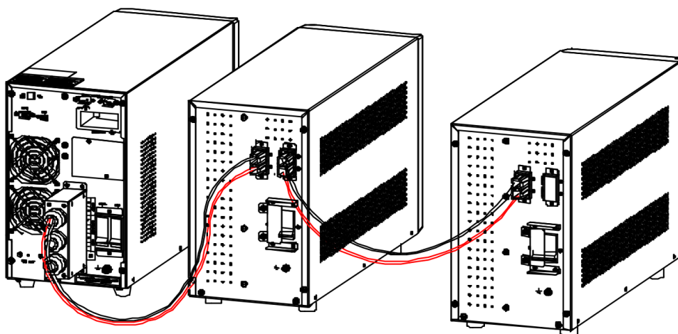
Подключение батарейных кабинетов к ИБП
