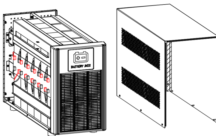
Расположение аккумуляторных батарей внутри батарейного кабинета
